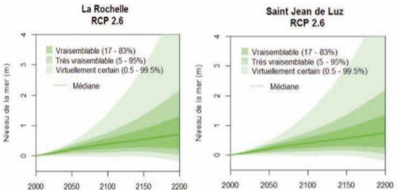
PROJECTION D'ÉLEVATION DU NIVEAU DE LA MER D'APRES L'ÉTUDE DE KOPP ET AL. (12) SOURCE : RAPPORT ACCLIMATERRA 2018
