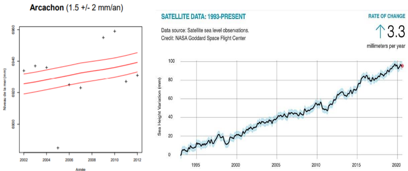
ELEVATION DU NIVEAU DE LA MER A ARCACHON ENTRE 2002 ET 2012 (DONNEES DREAL GPM BORDEAUX) ET COMPARAISON AVEC L'ELEVATION GLOBALE DU NIVEAU MARIN ENTRE 1995 ET 2020 (DONNEES SATELLITAIRES NASA)
